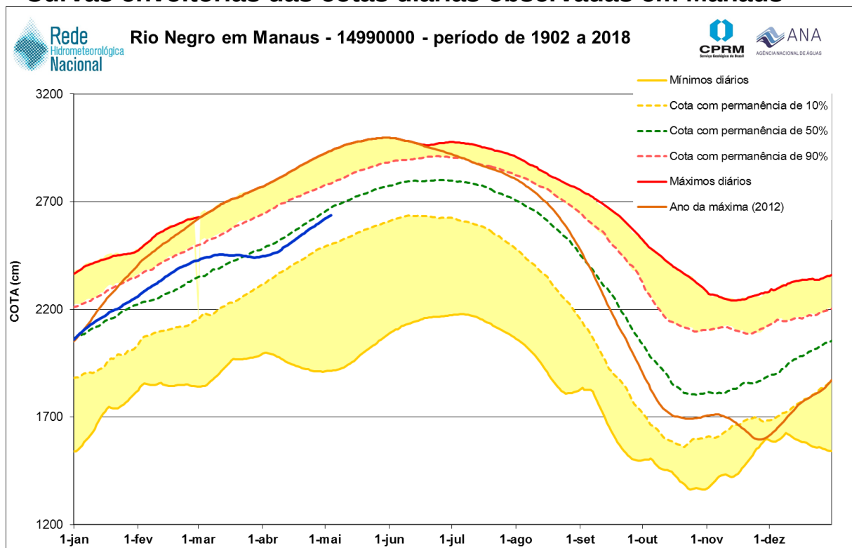
Gráfico 01: Cotograma do Rio Negro em Manaus. Cota em 11/05/2018: 26,86 m
